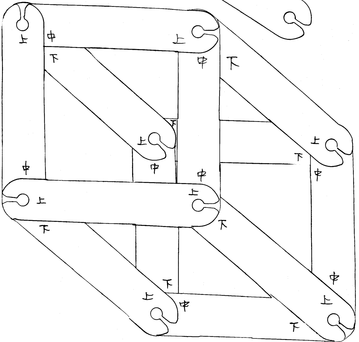
立方体組立圖
